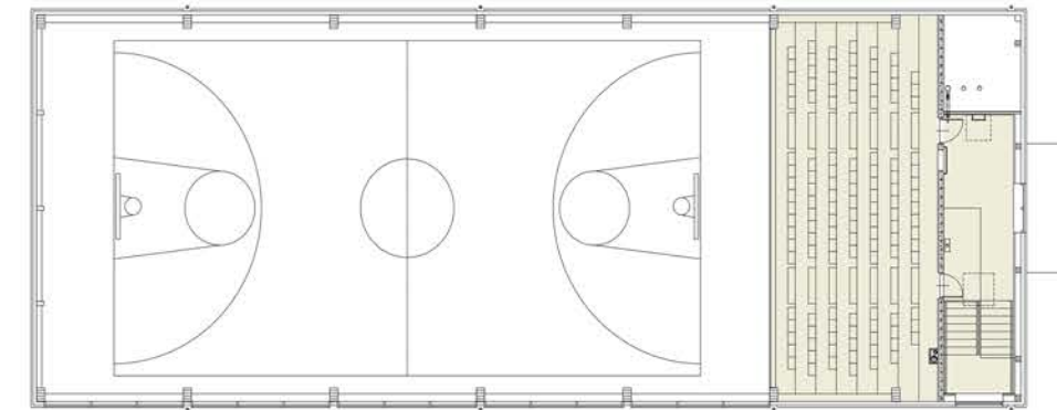
RZUT PIĘTRA
