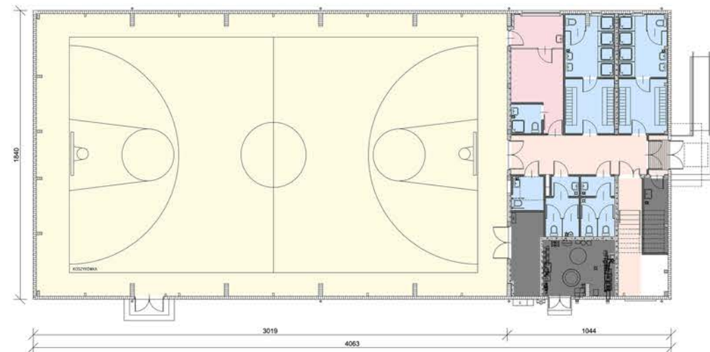
RZUT PARTERU
