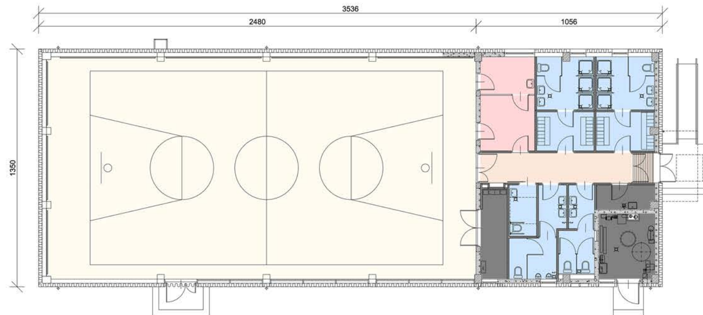
RZUT PARTERU
