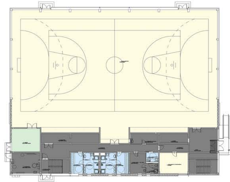
RZUT PARTERU
