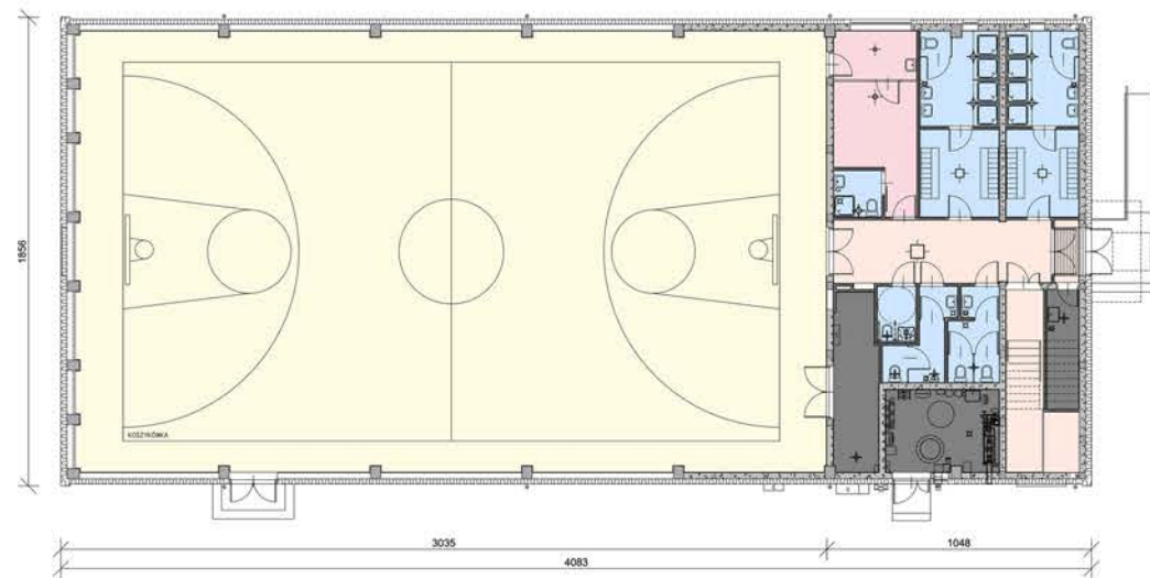
RZUT PARTERU
