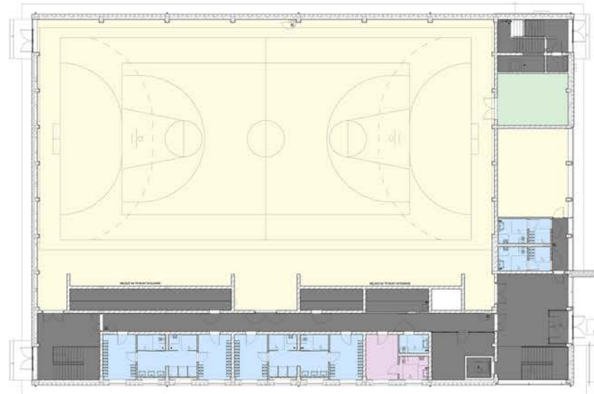
RZUT PARTERU
