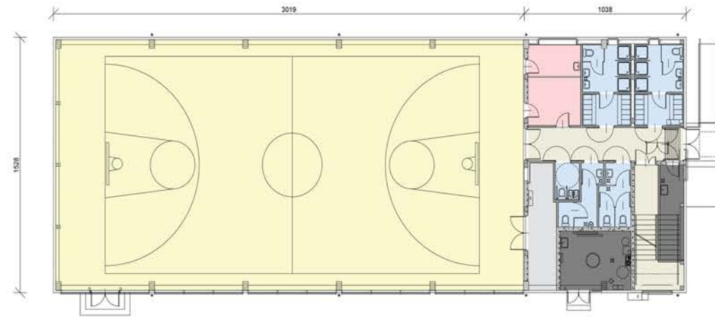
RZUT PARTERU
