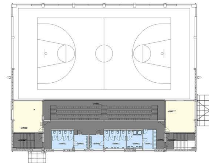
RZUT PIĘTRA
