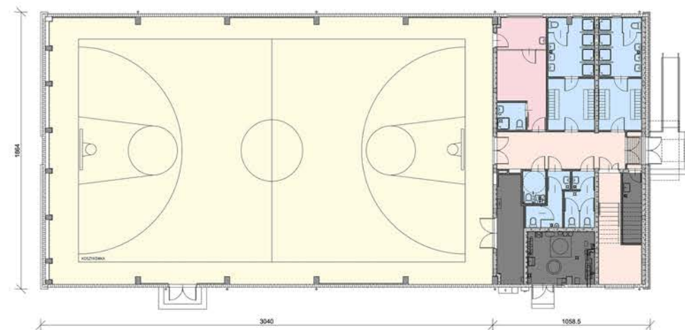
RZUT PARTERU
